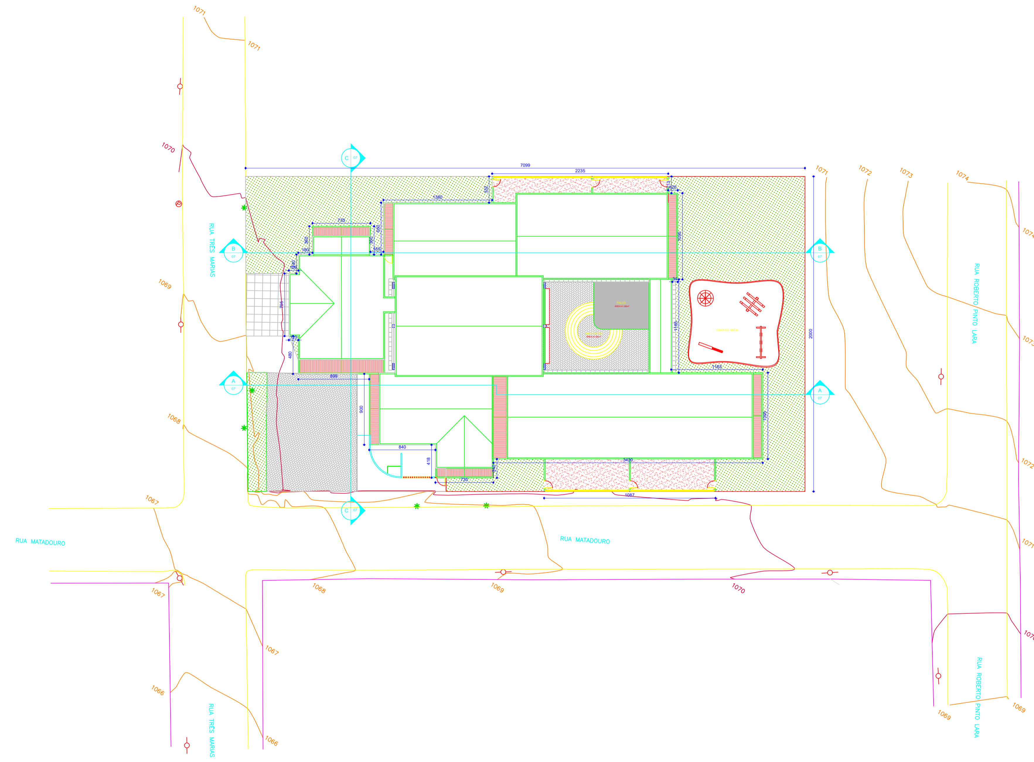
PLANTA DE IMPLANTAÇÃO ESC. 1:200
