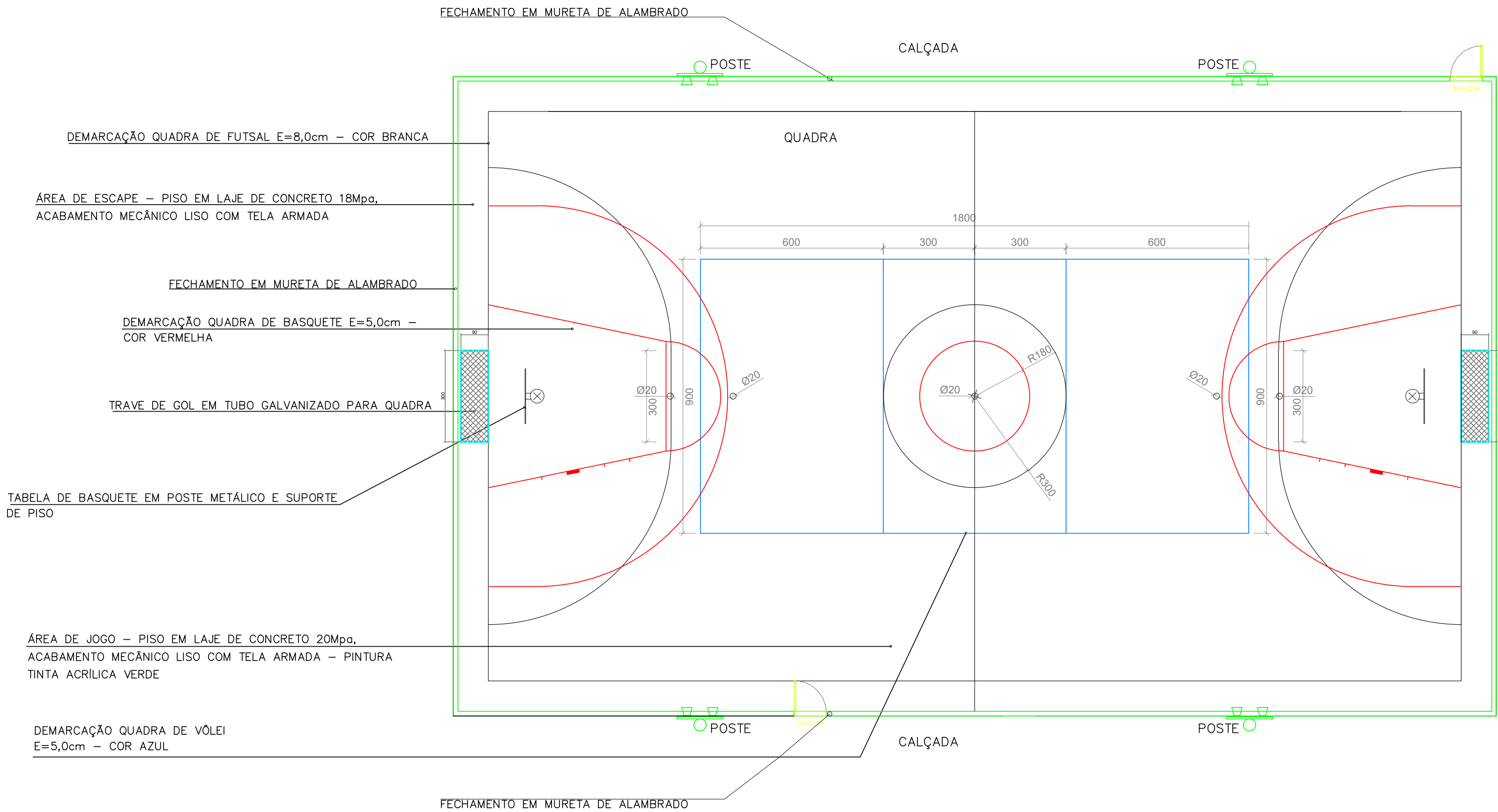
PLANTA DEMARCAÇÃO DA QUADRA ESC. 1:100
