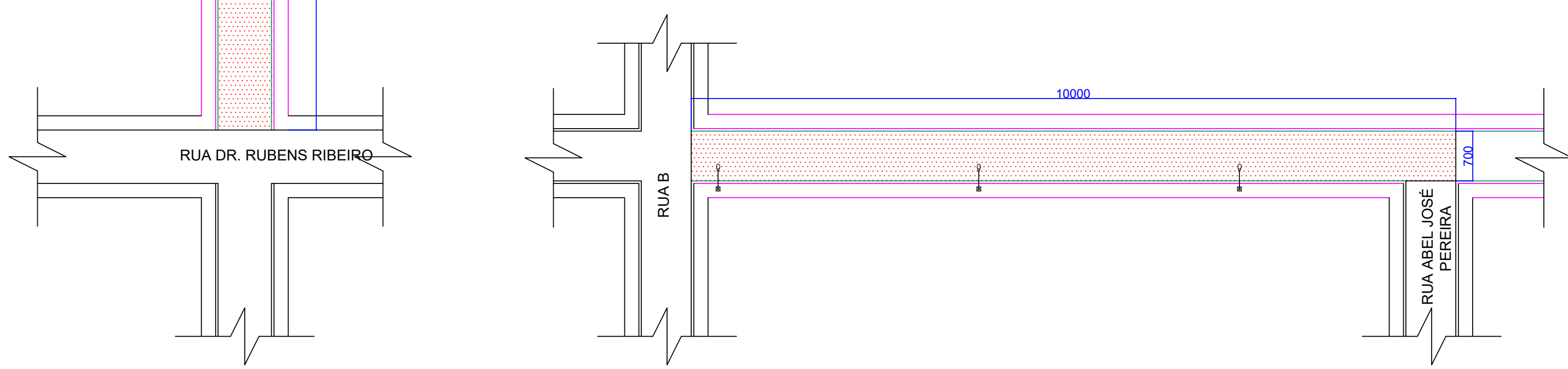
PAVIMENTAÇÃO EM CBUQ RUA DR. RUBENS RIBEIRO ESC. 1:500
