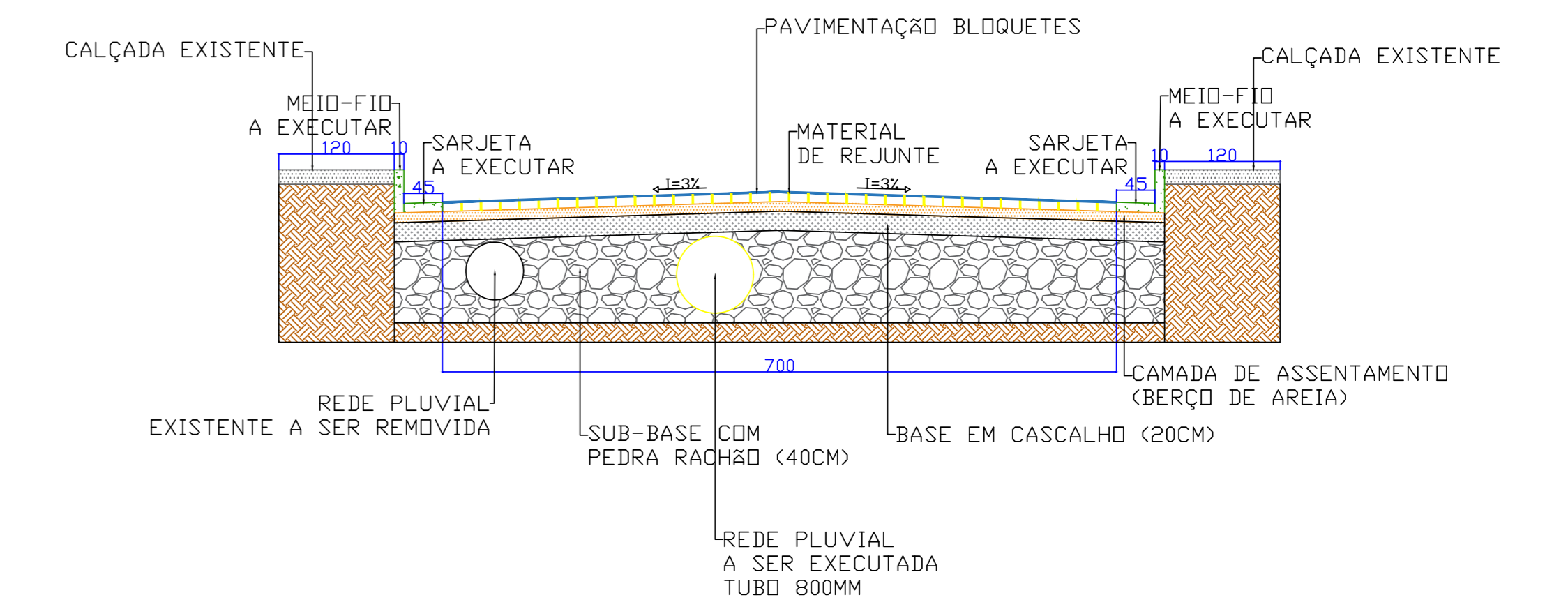
CORTE TRANSVERSAL RUA VITORINO VAGNER ESC. 1:50
